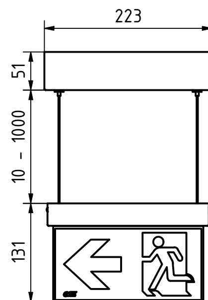
ASKELLA 20 Z DA-Seil
