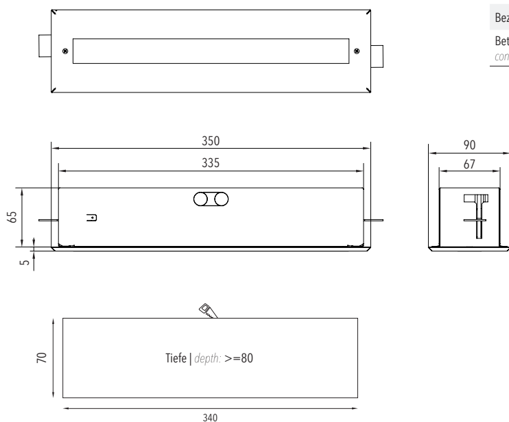
Ausschnitt für Wand- und Deckeneinbau section for wall and ceiling installation
