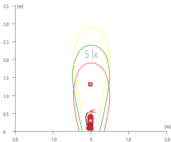
Montagehöhe der Leuchte | Mounting height of the luminaire — 2,0 m — 2,5 m — 3,0 m
