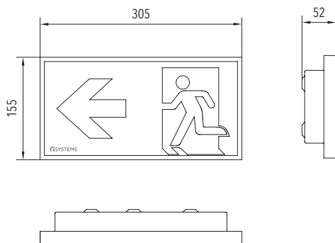
Wandaufbau (WA) wall mounting (WA)
